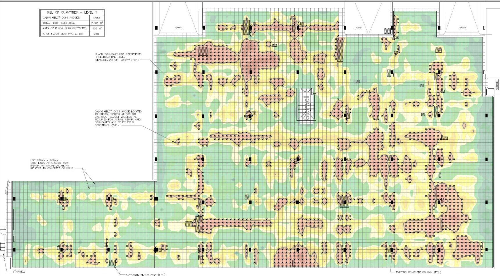
LEVEL 5 HALF-CELL POTENTIAL MAP & GALVANIC ANODE LAYOUT SCALE: N.T.S.
